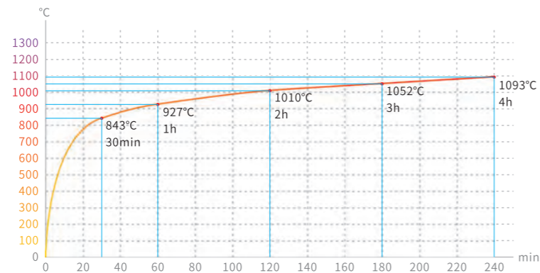
美国UL-72 外部时间温度测试标准曲线
